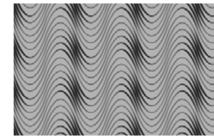
M14
