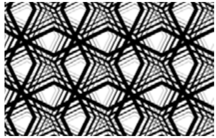
M25
