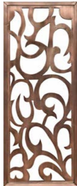
M101
