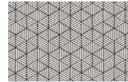
M20
