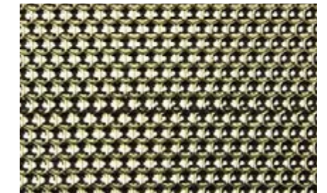
M78
