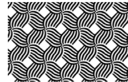
M16
