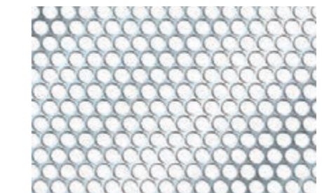
M60
