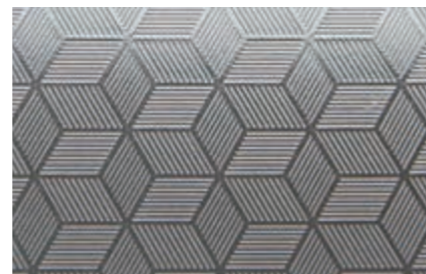
M51
