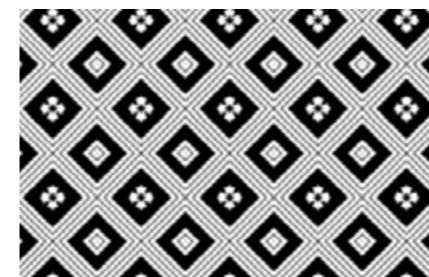
M40
