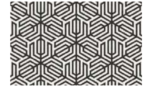
M21
