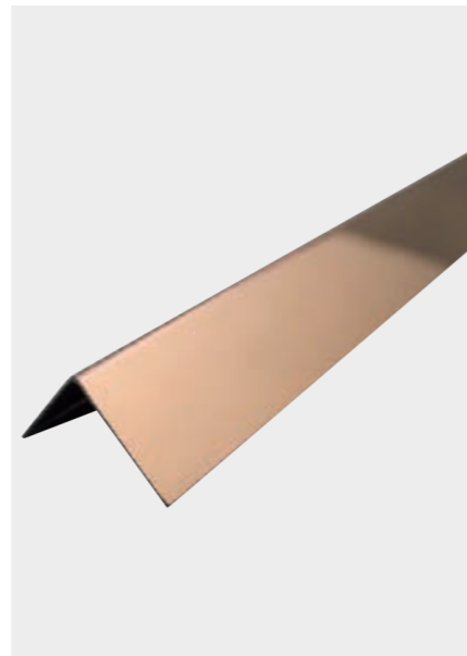
M109
