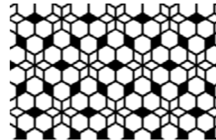
M37
