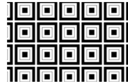
M38
