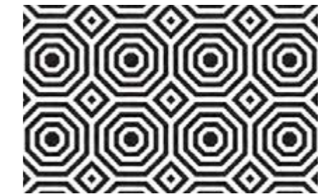
M15
