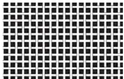
M34
