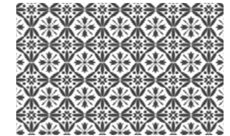
M24
