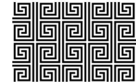
M39
