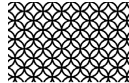
M23
