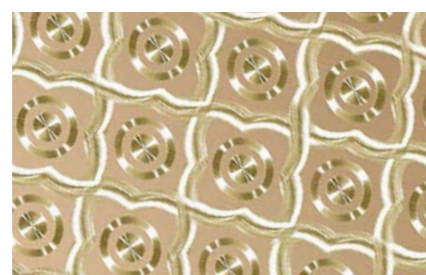
M71
