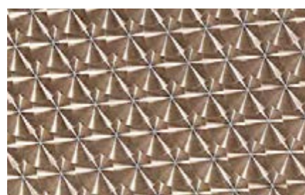
M70
