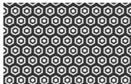
M35
