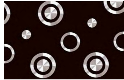
M63
