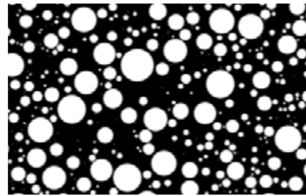
M29
