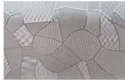
M45
